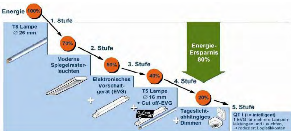
Abbildung 25: Einsparpotential Beleuchtung 24
