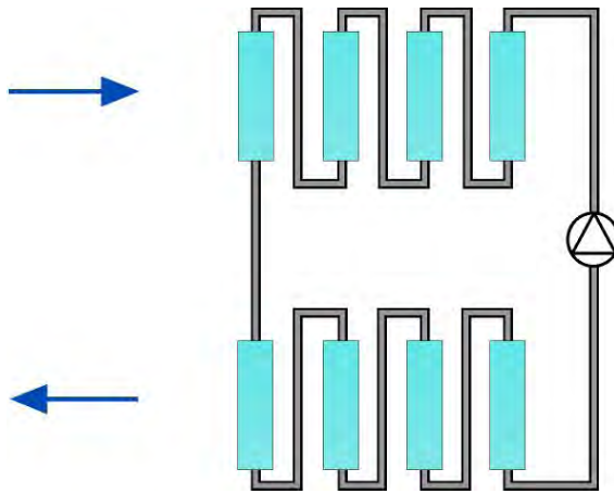
Abbildung 23: Kreislaufverbund Wärmetauscher 20
